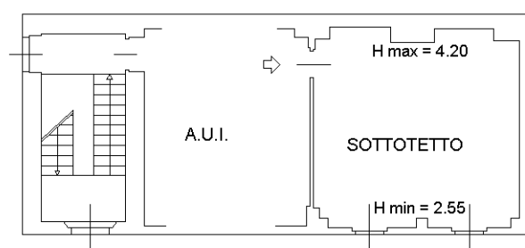
PIANO SOTTOTETTO
