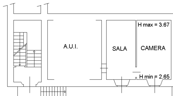
PIANO PRIMO
